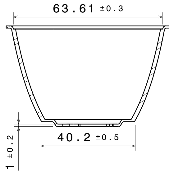
Section view A-A Scale: 1:1
