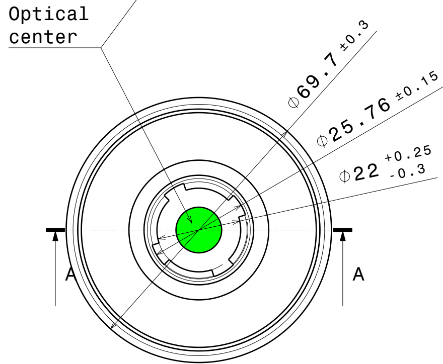
Top View Scale: 1:1
